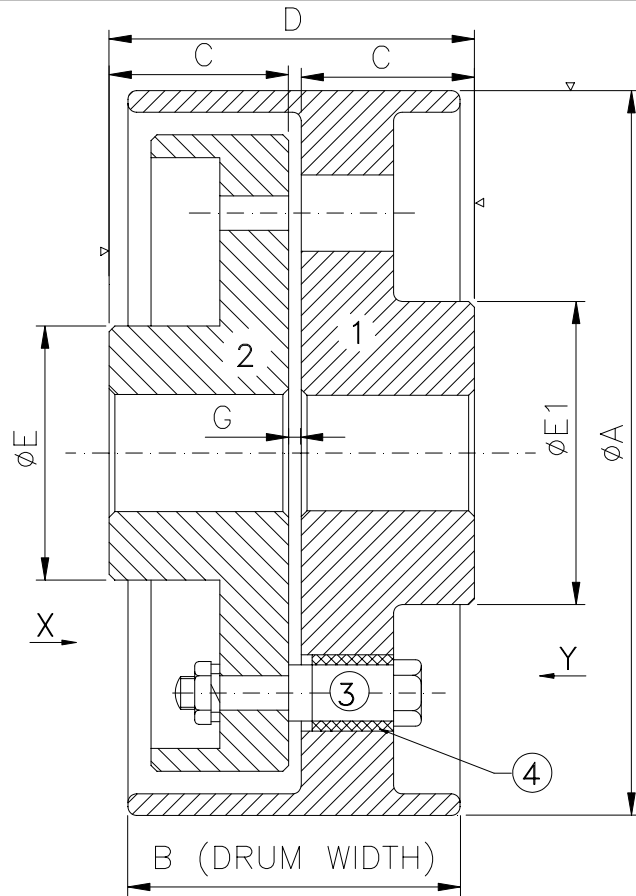
DIMENSIONS
